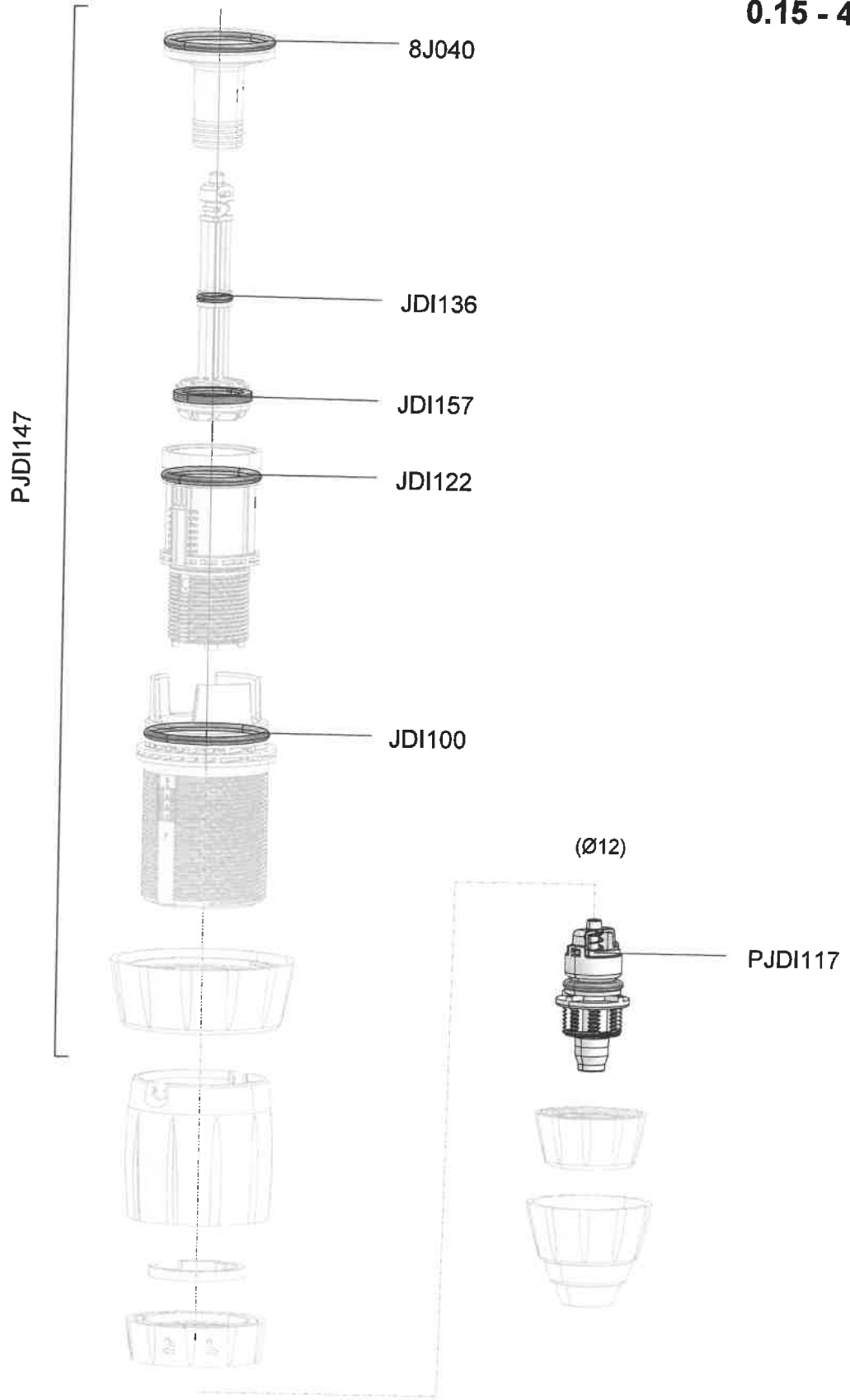
Seal Kit - PJD1147 (8J040, JDI136, JDI157, JDI122, JDI100, PJD1117)
